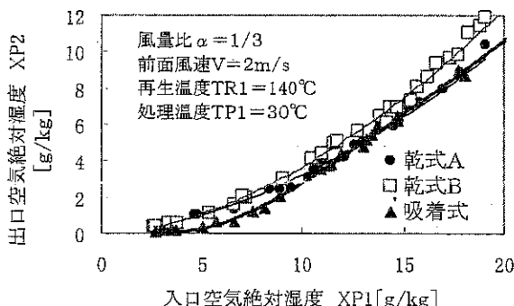
図3 除湿性能比較
