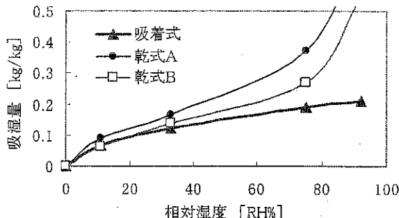
図2 平衡吸湿量の比較
