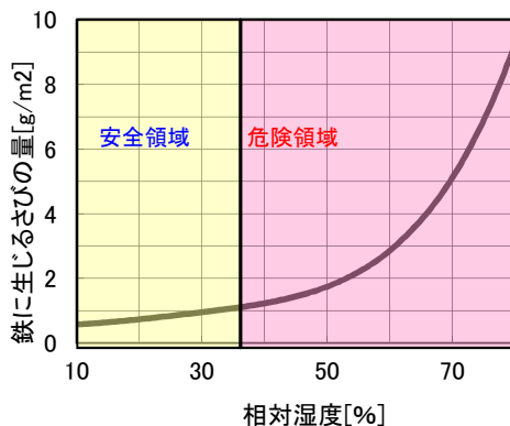
さびの発生量と相対湿度
